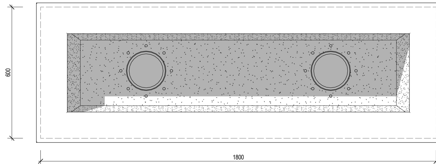
3 PLAN 001 1 : 10 @ A3
