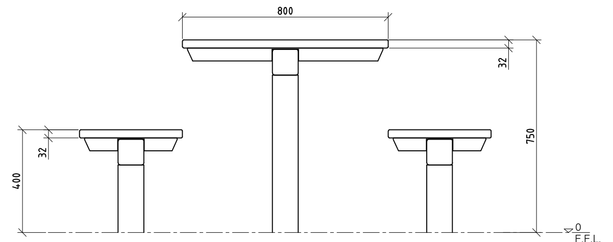
3 END ELEVATION 1:15 @ A3
