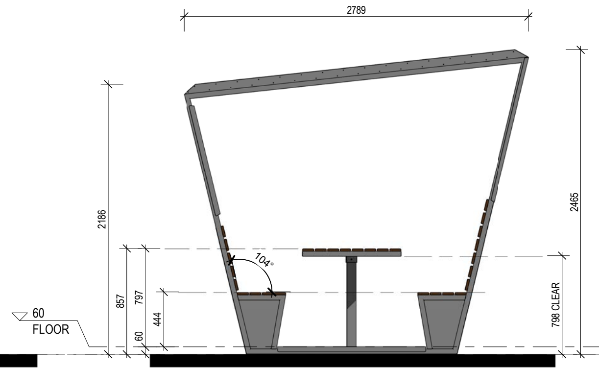
2 ELEVATION 1 001 1:30 @ A3
