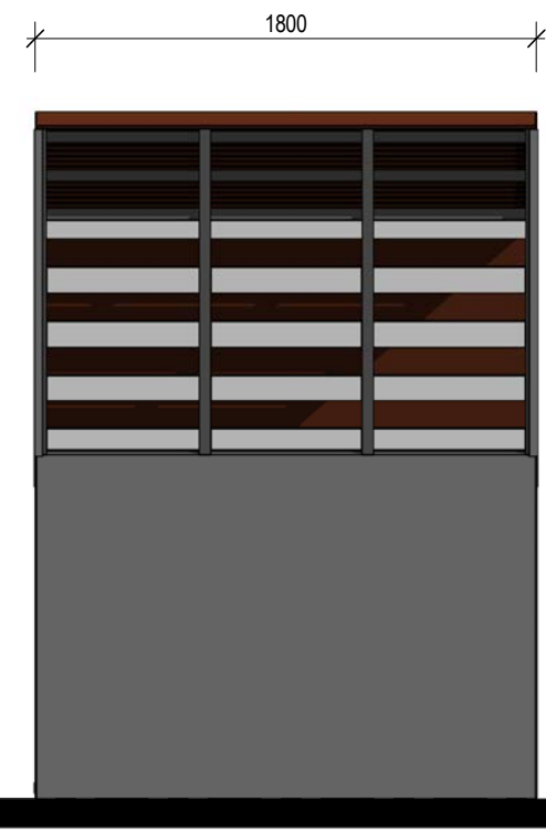
3 ELEVATION 2 001 1:30 @ A3
