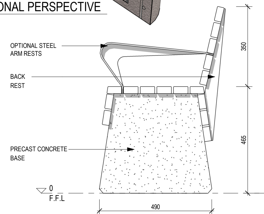
4 END ELEVATION 1 : 10 @ A3
