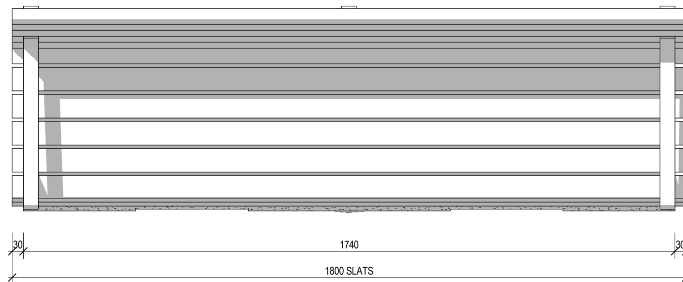
3 PLAN 001 1 : 10 @ A3
