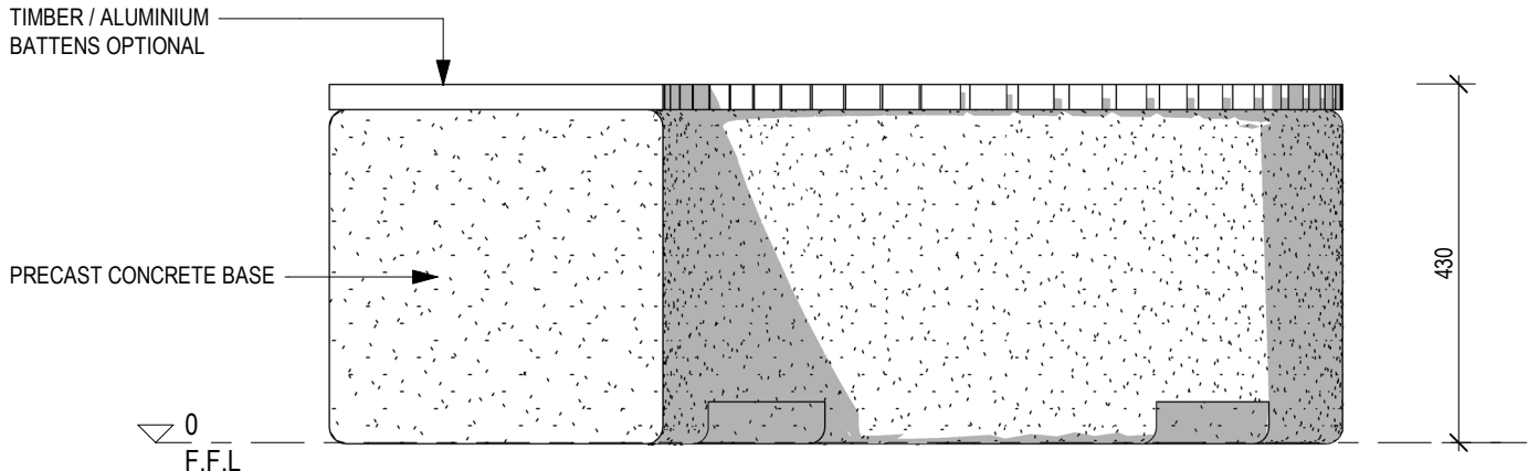
4 END ELEVATION 1 : 10 @ A3
