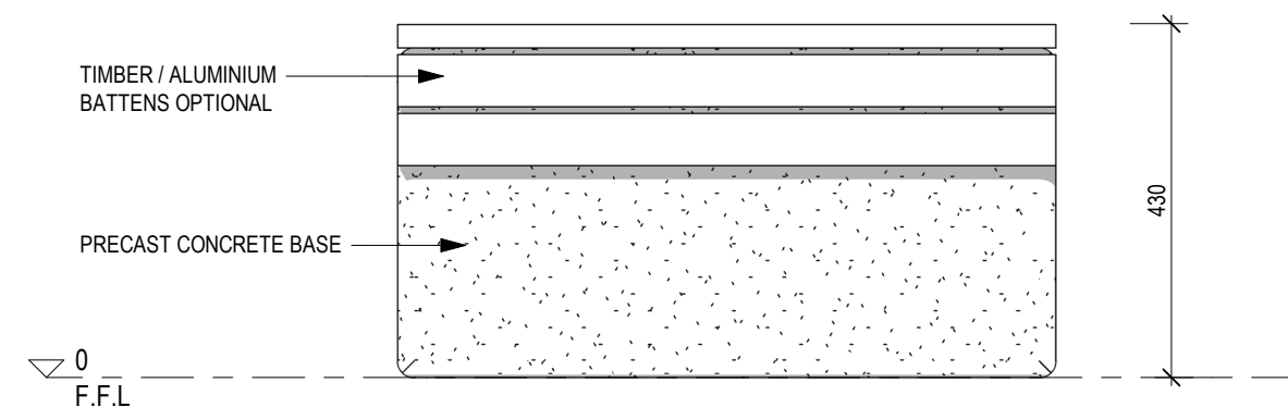
4 END ELEVATION 1:10 @ A3
