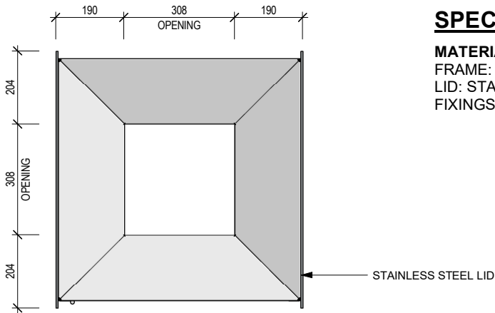
4 SECTION 1 : 15 @ A3
