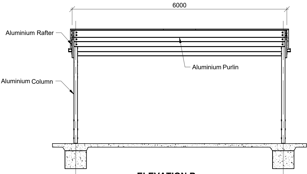
ELEVATION B 1:50
