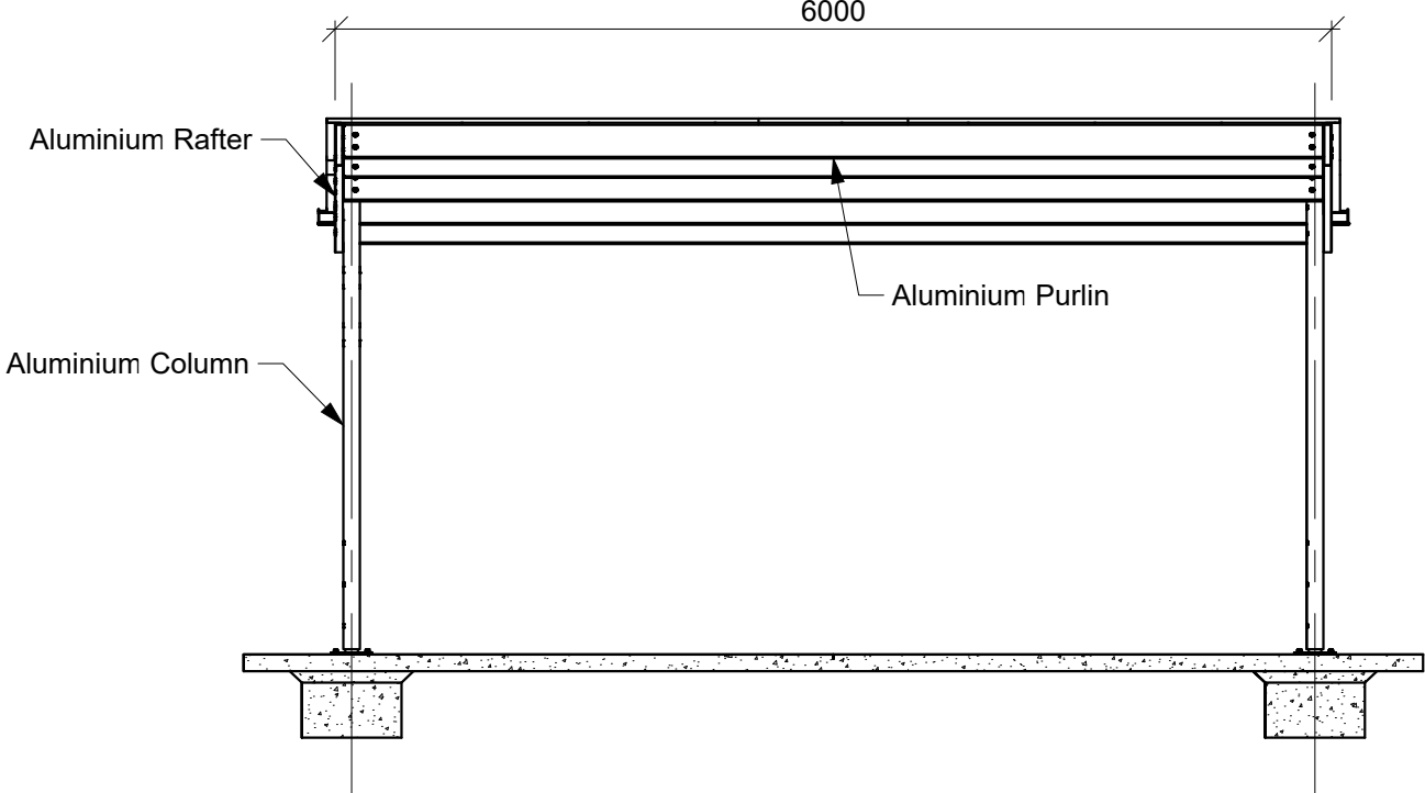
ELEVATION B 1:50
