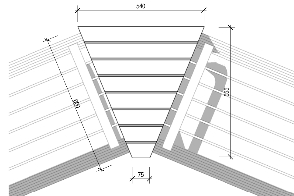
5 PLAN 1:10 @ A3
