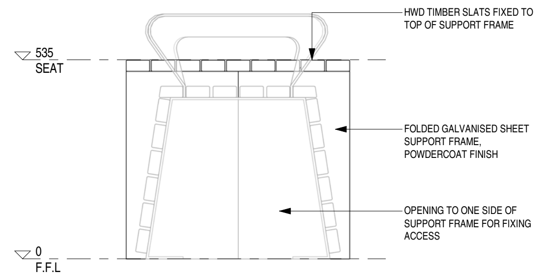
2 END ELEVATION 1:10 @ A3
