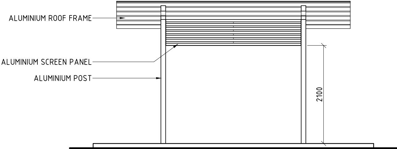
ELEVATION E1 SCALE (1:50) 101
