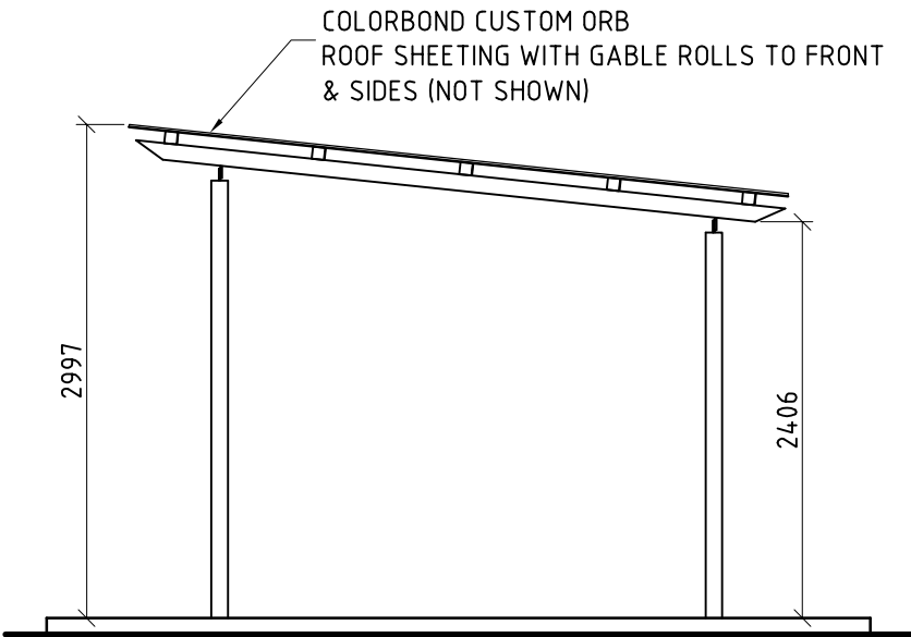
ELEVATION E2 SCALE (1:50) 101
